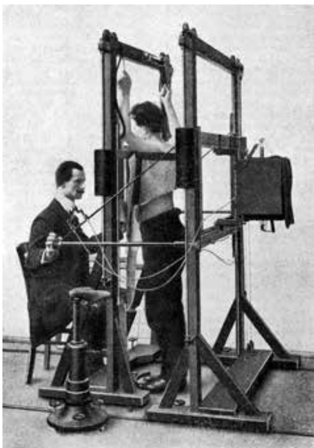
Afb. 43 Het Groninger statief, ontwikkeld door Wenckebach en zijn amanuaensis Bootsgezel, om stereografische röntgenafbeeldingen te krijgen. Uit: Nederlandsch Tijdschrift voor Geneeskunde (1910) IIB, 1396.
