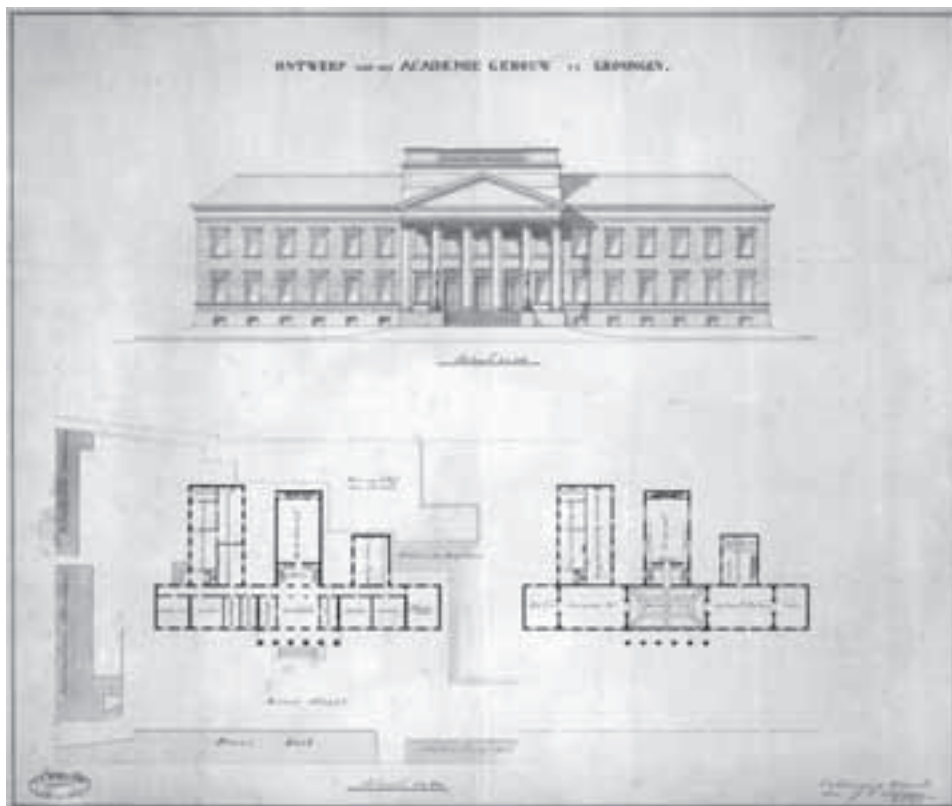
Afb. 96 Vooraanzicht en plattegrond van beneden- en bovenverdieping van het in 1850 gereedgekomen Academiegebouw. Bestektekening uit 1849. RHC Groninger Archieven.
