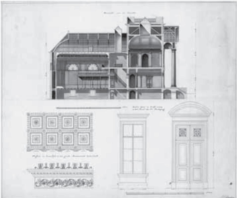
Afb. 95 Bestektekening van het nieuwe Academiegebouw, door J.F. Scheepers, 1846. RHC Groninger Archieven.
